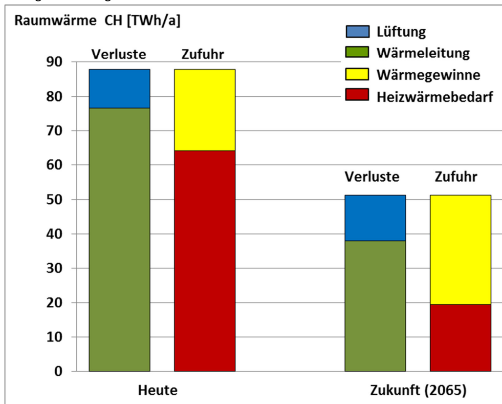
Abbildung 10: Heizwärmebilanzen des gesamten Gebäudebestandes der Schweiz, heute und in 50 Jahren
